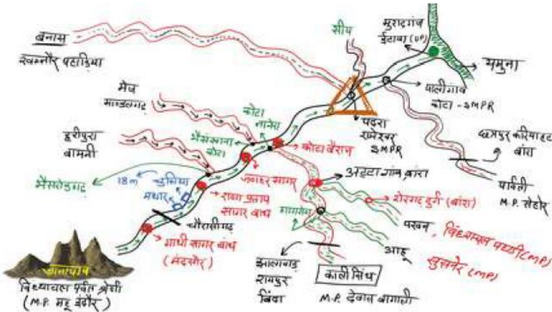
चित्र 4.3 : चम्बल, कि सायक नदियों का उद्गम
